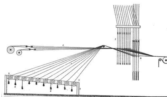
Fig 2 : Cantre vue par le côté
