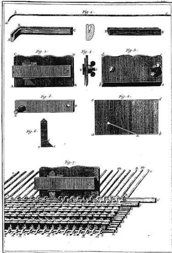
Soterie, Velours Coupé. Fers de Coupé, Rabot—, m m m Trillerolle: Usage du Rabot et Velours Coupé Vu au Microscope et en perspective.
