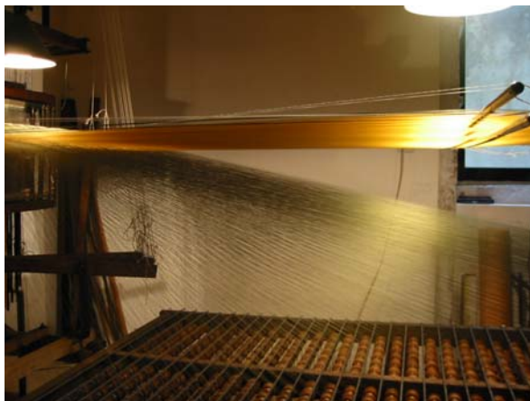
Les fils poil remontent de la cantré à velours. Atelier Agnès Alauzet
