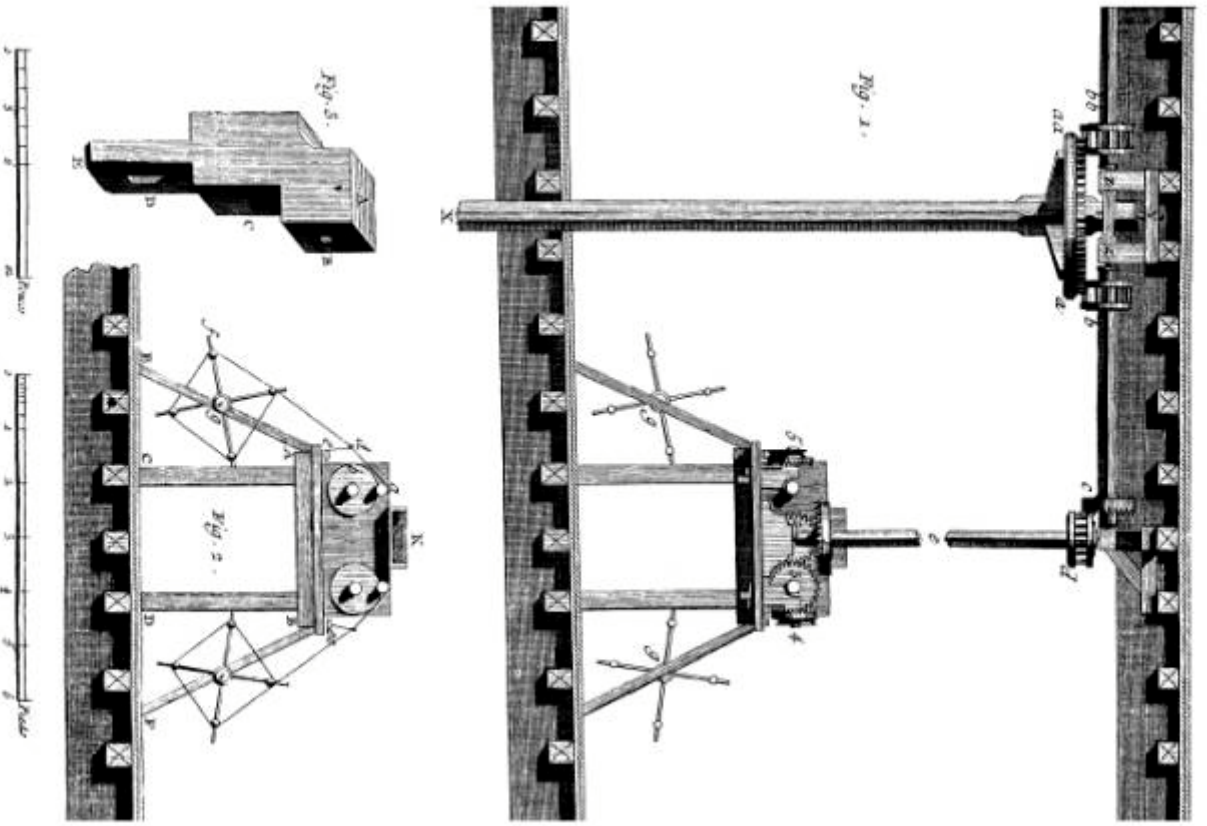
Soierie, Profil du Dessilage qui est en haut des Moteurs à l'égouttoir de soie
