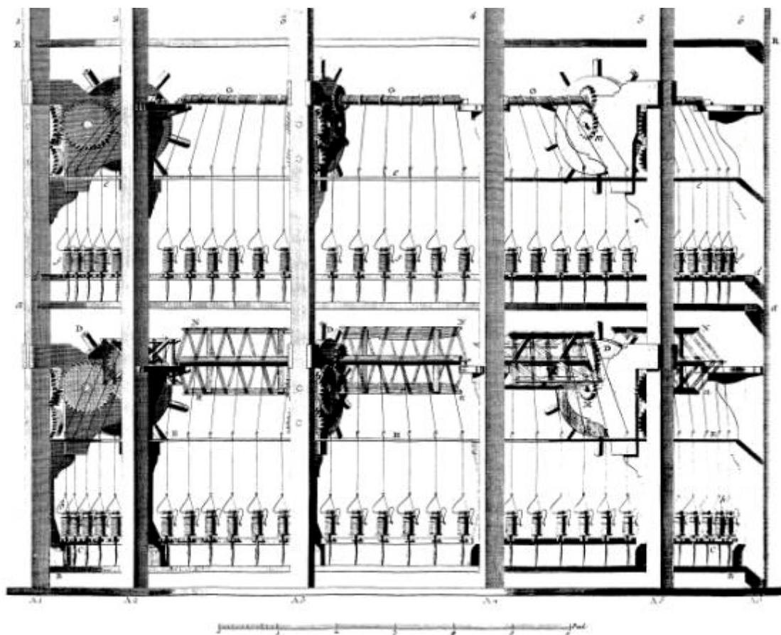
Soierie, Elevation Géométrale du Moulin de Pérou, pour Organiser les Cages.
