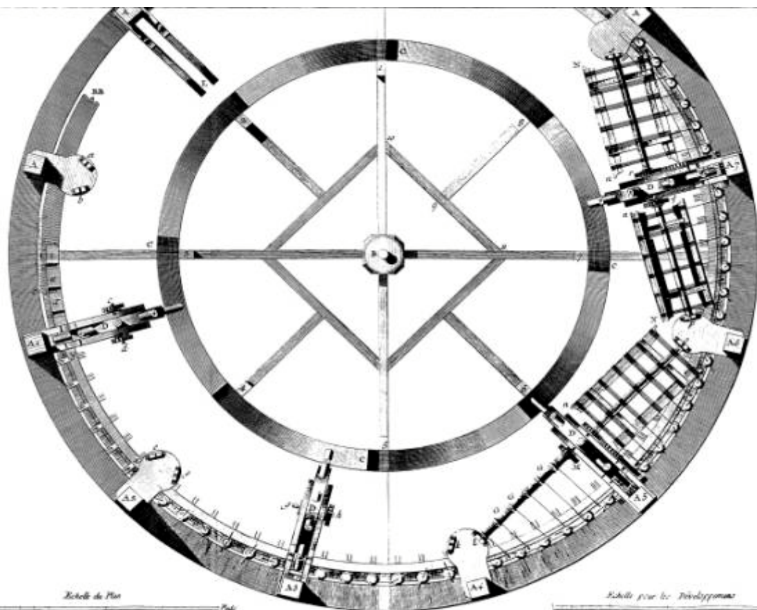
Soierie, Plan du Moulin de Pérouse, à Strassbourg pour Organiser les Soies.
