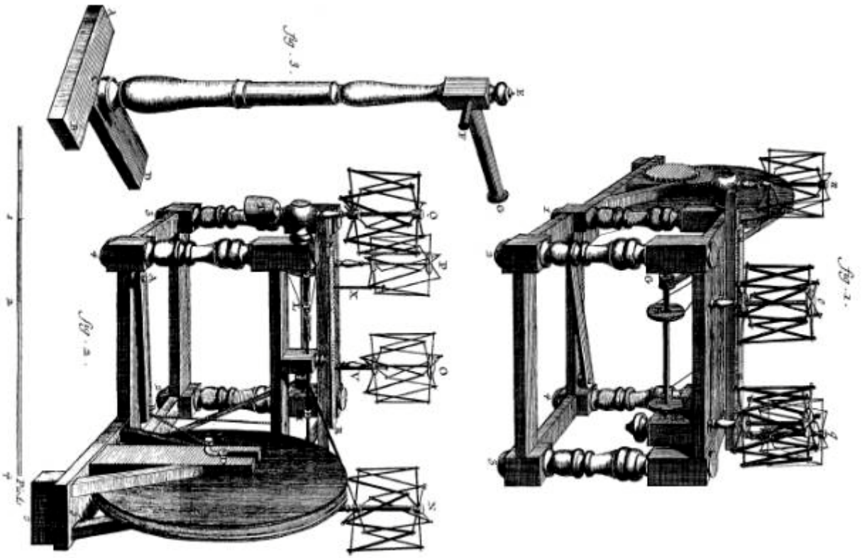
Soierie, Rouet de Lion ou Perceuse vu des deux côtés.
