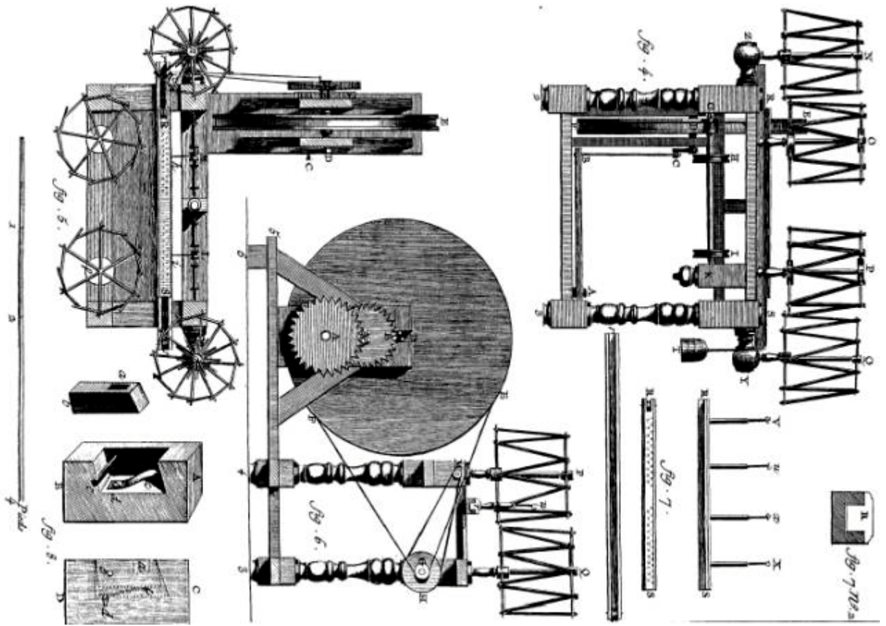
Soierie, Rouet de Lion, Développement.
