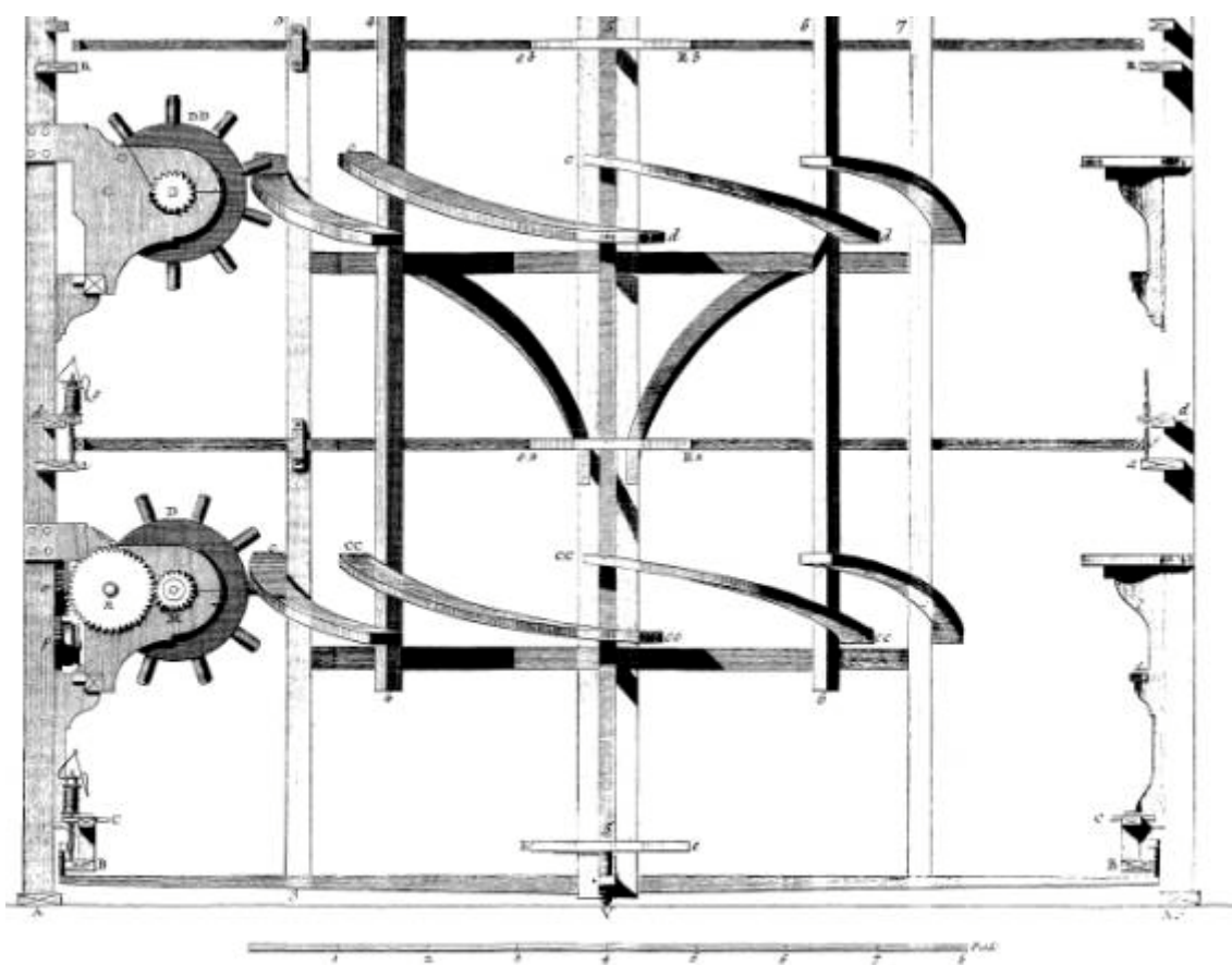
Soierie, Coupe Diamétrale du Moulin de Pérou et Elevation de la Lanterne qui est dans l'Intérieur.
