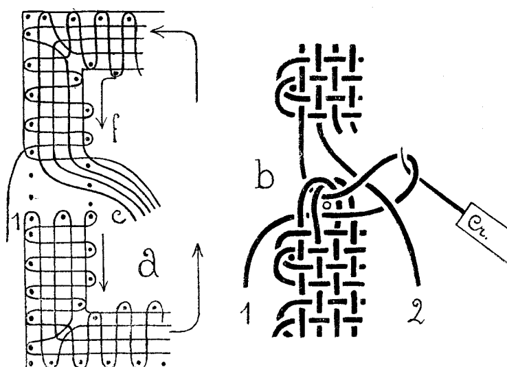
Fig. 71. — Terminaison du galon : la fin f doit être fixée au commencement c . En b , détail d'un accrochage.
