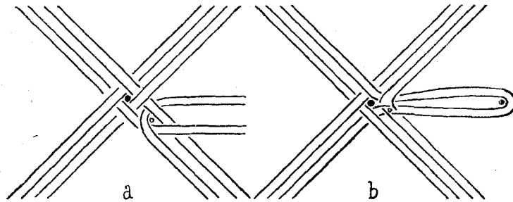
Fig. 24. — Bride de 2 fils fixée à un croisement de 2 tresses.
