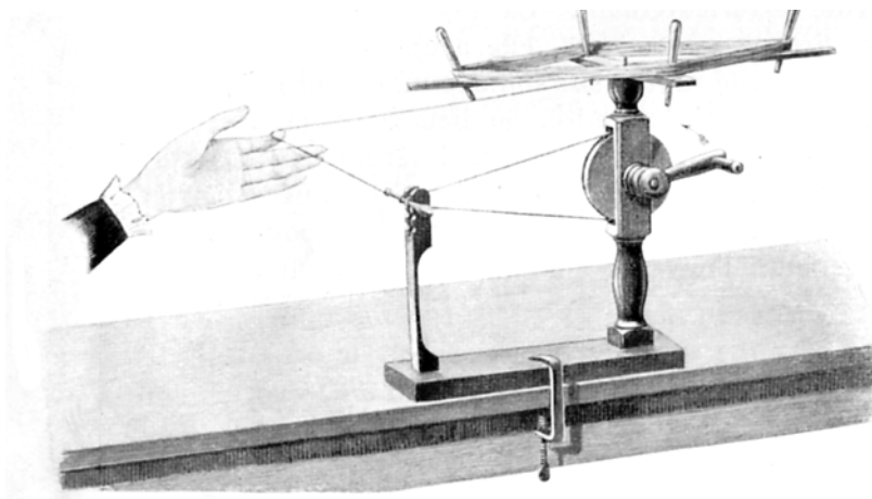
Fig. 4. Le bobinoir.
